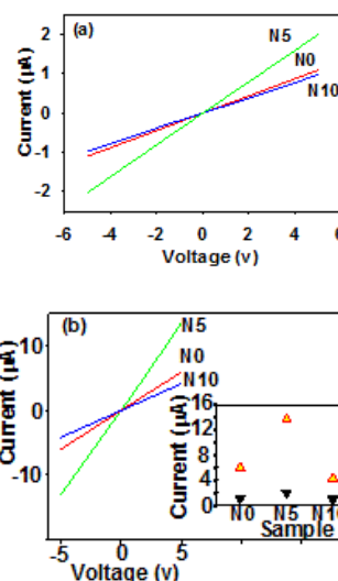
شکل ۵: مشخصه جریان-ولتاژ نمونه های مورد بررسی در شرایط (الف) تاریکی و (ب) تحت تابش نور UV. شکل ضمیمه تغییرات جریان نوری را برای نمونه های سنتر شده نشان می دهد. در این شکل علائم \blacktriangledown مربوط به شرایط تاریکی و علائم \blacktriangle مربوط به شرایط نور تابی است.
