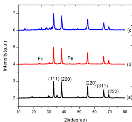
شکل ۱: الگوی پراش پرتو ایکس. (a) اکسید کادمیم بدون آلیاژ - (b) اکسید کادمیم ۵٪ آلیاژ شده با آهن - (c) اکسید کادمیم ۱٪ آلیاژ شده با آهن
