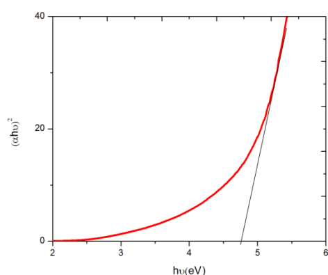
شکل ۲-ب (۳): گاف انرژی اکسید کادمیم ۱٪ آلاینده شده با آهن
