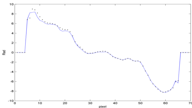
شکل ۸: نمودار خط چین نشان دهنده سطر ۳۰ مربوط به اختلاف فاز بازسازی شده (اختلاف شکلهای ۶ و ۷) و نمودار توپر اختلاف فاز دو باریکه که با روش انتقال فاز به دست آمده است. محور افقی شماره پیکسلها و محور عمودی بر حسب رادیان می‌باشد.
