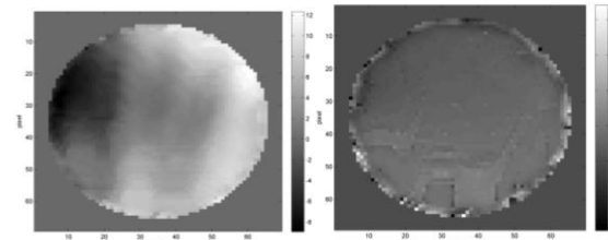
شکل ۶: فاز بازسازی شده برای باریکه اول (سمت راست) و باریکه دوم (سمت چپ) بر حسب رادیان.
