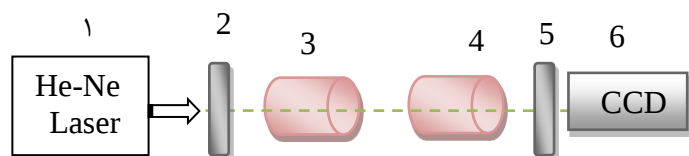
شکل ۲: چیدمان قطبش نگاری، لیزر هلیوم نئون موازی شده، ۲ و ۵ قطبنده و واكافنده، ۳ و ۴ میله لیزر Nd:YAG، ۶: CCD
