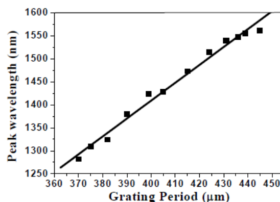
شکل ۷: نمودار مربوط به توری گام‌بلند ایجاد شده بر روی یک موجبر پلیمری [7].
