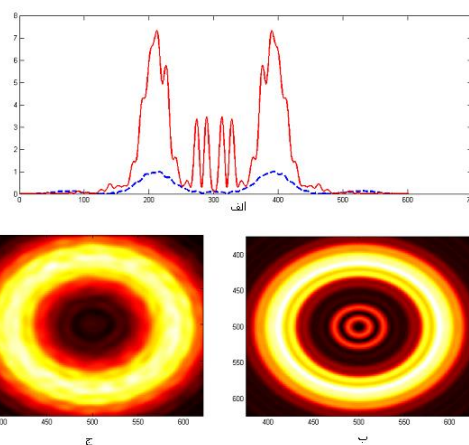
شکل ۷-الف- نمودار با رنگ قرمز از نمونه پیرایش نشده و نمودار آبی از نمونه پیرایش شده بدست آمده. ب- شدت شبیه سازی شده برای حالت پیرایش نشده. ج- شدت شبیه سازی شده برای حالت پیرایش شده
