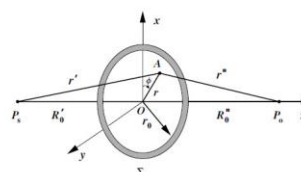
شکل ۱- پراش از روزنه حلقه ای
