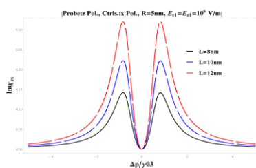
شکل ۴: نمودار قسمت موهومی پذیرفتاری الکتریکی یک نقطه کوانتومی استوانه‌ای با ارتفاع‌های متفاوت در میدان کاوشگر با قطبش Z (الف) میدان کنترل با قطبش Z (ب) میدان کنترل با قطبش X (الف)
