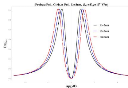
شکل ۵: نمودار قسمت موهومی پذیرفتاری الکتریکی یک نقطه کوانتومی استوانه‌ای با شعاع‌های متفاوت در میدان کاوشگر با قطبش Z (الف) میدان کنترل با قطبش Z (ب) میدان کنترل با قطبش X (الف)
