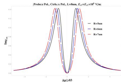
شکل ۵: نمودار قسمت موهومی پذیرفتاری الکتریکی یک نقطه کوانتومی استوانه‌ای با شعاع‌های متفاوت در میدان کاوشگر با قطبش Z (الف) میدان کنترل با قطبش Z (ب) میدان کنترل با قطبش X (الف)
