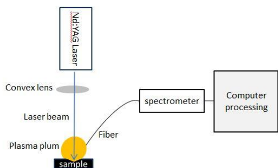
شکل ۱: طرحواره چیدمان آزمایش
