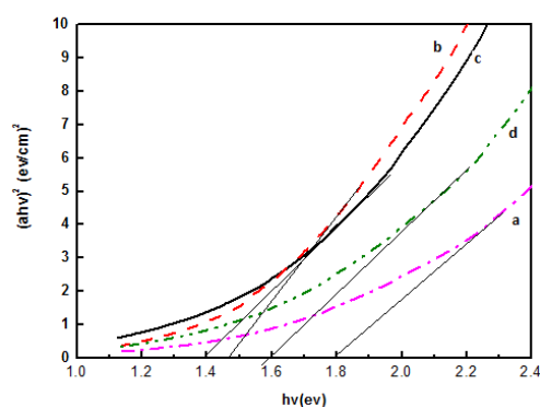
شکل ۳- نمودار Tauc برای نانو ذرات Pb_{1-x}Sn_xS به ازای مقادیر (a) x=0 ، (b) x=0.02 ، (c) x=0.05 ، (d) x=0.1 [۸]
