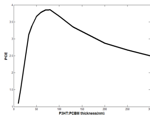
شکل ۲: منحنی بازده بر حسب تغییرات ضخامت لایه فعال
