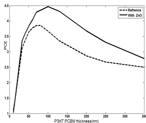
شکل ۵: منحنی بازده دو OSC برحسب ضخامت لایه فعال
