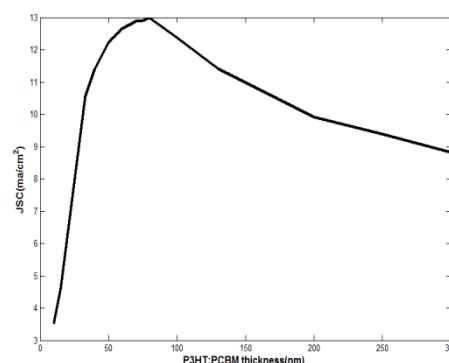
شکل ۳: منحنی چگالی جریان بر حسب ضخامت لایه فعال
