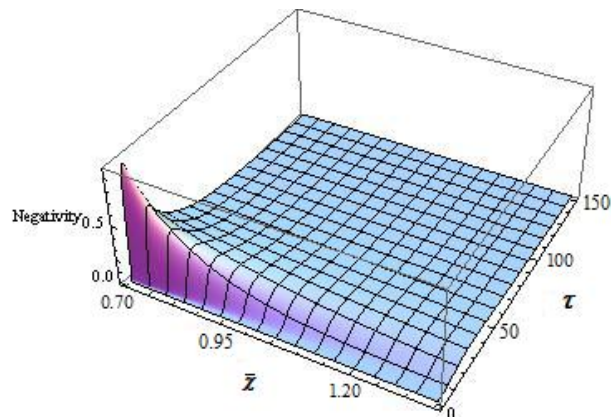
شکل ۴: نمودار سه بعدی درهمتیدگی براساس دما و عامل غیرخطی دگرکنش.
