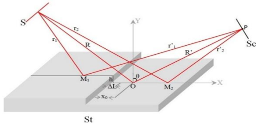
شکل ۱: شمای پراش فرنل از پله فازی. S چشمه خطی به موازات لبه پله و St ، پله و Sc پرده مشاهده عمود بر باریکه بازتابیده است.
