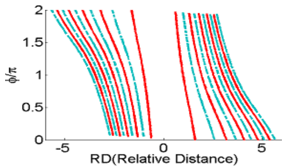
شکل ۳: نمودار تغییرات فاز بر حسب کمیت RD برای پنج بیشینه و پنج کمینه اول سمت راست لبه پله (که مقادیر RD برای این فرینه‌ها مثبت است) و همچنین برای سمت چپ لبه پله (که مقادیر RD برای آنها منفی است). خطوط پیوسته مربوط به بیشینه‌ها و خطوط گسسته مربوط به کمینه‌ها هستند.
