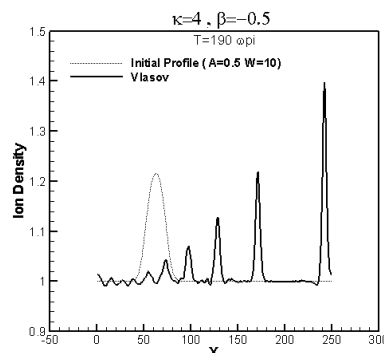
شکل ۲. تولید سالیتون از پروفایل اولیه با دامنه 0.5/0.5 از روش شبیه سازی
