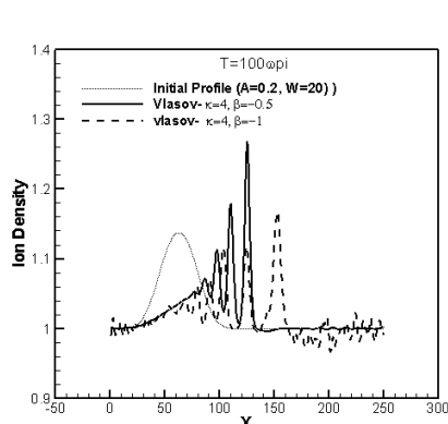
شکل ۴. تولید سالیتون با استفاده از روش شبیه سازی برای پروفایل اولیه با دامنه 0.5/2 به ازای مقادیر مختلف \beta
