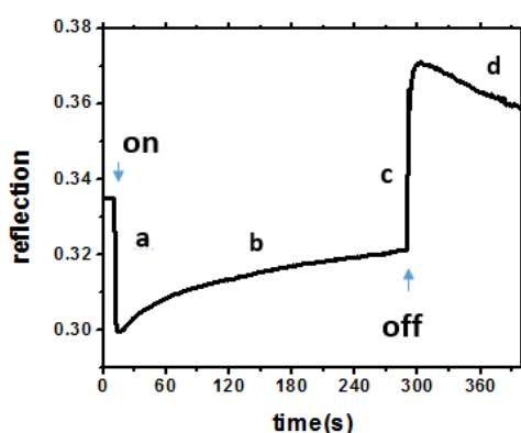
شکل ۴: نمودار بازتاب برحسب زمان برای رنگینه‌ی DO۲۵ با اعمال نور لیزر دمشی با توان ۲ میلی وات.
