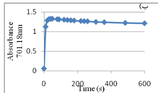
شکل ۱: الف) طیف جذبی نانوذرات طلا- پروپیل مرکاپتان در زمان ۰-۱۲۰۰ ثانیه. ب) نمودار جذب بر حسب زمان نانوذرات طلا- پروپیل مرکاپتان در طول موج ماکزیمم می‌باشد.
