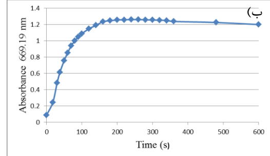
شکل ۲: الف) طیف جذبی نانوذرات طلا- پنتیل مرکاپتان در زمان ۰-۱۲۰۰ ثانیه. ب) نمودار جذب بر حسب زمان نانوذرات طلا- پروپیل مرکاپتان در طول موج ماکزیمم می‌باشد.
