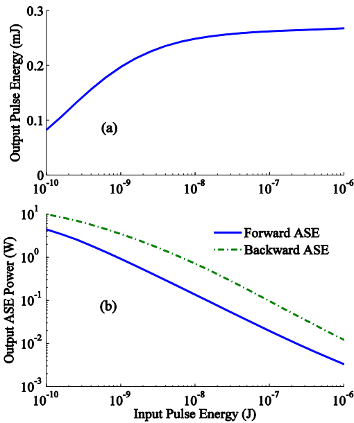
شکل ۵: نمودار (a) انرژی پالس خروجی تقویت‌کننده بر گسیل خود به خودی تقویت شده خروجی رو به جلو و رو به عقب، بر حسب انرژی پالس ورودی.
