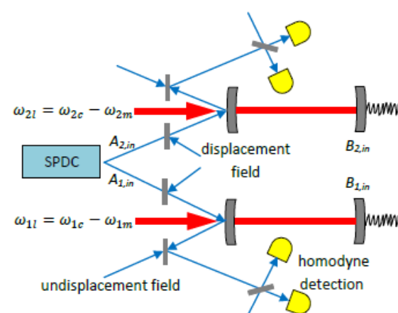
شکل ۱: سامانه ایجاد درهمتنیدگی میکرو-ماکرو بین پرتوهای فشرده درهمتنیده و کاواکهای اپتیک دور از هم که به صورت واکوکی قرمز راه اندازی شده اند [۲].
