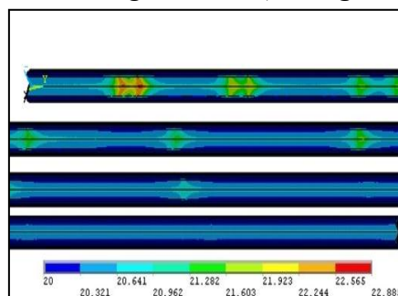
شکل ۷ گستره دمایی سیستم برای توان 200\text{W}
