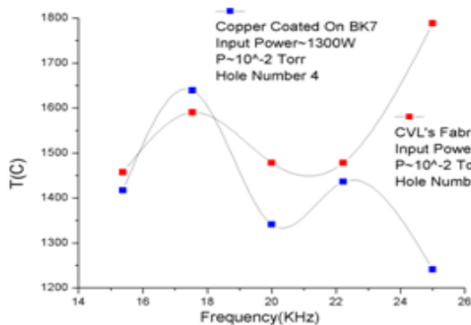
شکل ۴: قرمز: دمای دیواره لیزر بخار مس با آینه اصلی لیزر در فشار 10^{-2} Torr و با فرکانس‌های مختلف. آبی: دمای لیزر بخار مس با آینه مسی و زیر لایه BK7 در فشار 10^{-2} Torr در همان فرکانس‌ها.
