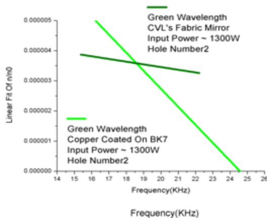
شکل ۶: نمودار فرکانس بر حسب n/n_0 برای طول موج سبز روزنه دوم در فشار 10^{-2} Torr و توان ورودی حدود ۱۳۰۰ W.
