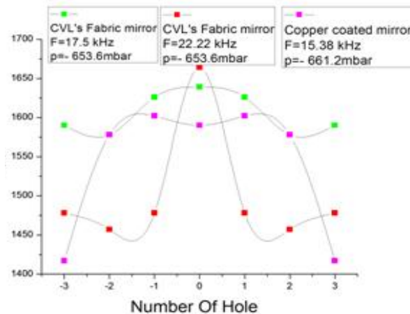
شکل ۳: قرمز: نمایه دمایی لیزر بخار مس با آینه اصلی لیزر در فرکانس ۲۲.۲ kHz در فشار 10^{-2} Torr؛ سبز: فرکانس ۱۷.۵ kHz در فشار 10^{-2} Torr؛ بنفش: نمایه دمایی لیزر با آینه مسی در فرکانس ۱۵.۳۸ kHz در فشار 10^{-2} Torr.
