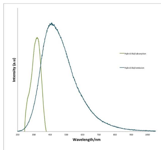
شکل ۱: منحنی جذب و انتشار نانوساختارهای \text{Alq}_3 .
