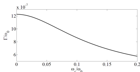
شکل ۱: نحوه تغییرات آهنگ رشد نرمالیزه در پراکندگی بریلوئن رو به جلو نسبت به فرکانس سیکلوترونی نرمالیزه.
