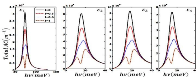
شکل ۴. نمودار ضریب جذب کل به صورت تابعی از انرژی فوتون های ورودی و به ازای مقادیر متفاوت شدت فوتون های تابشی در حضور ناخالصی هیدروژنی برای L = 8 nm و x = 0.3 .
