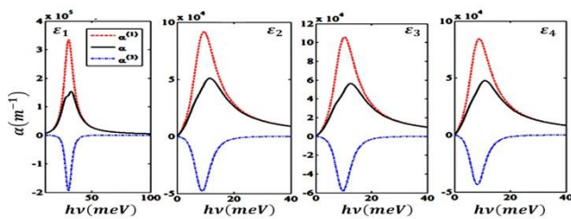
شکل ۳. نمودارهای ضریب جذب خطی، مرتبه سوم غیر خطی و ضریب جذب کلی به صورت تابعی از انرژی فوتون تابشی در حضور ناخالصی هیدروژنی و به ازای توابع استتار متفاوت، L = 8 nm و x = 0.15 .
