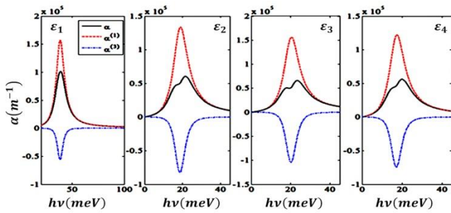
شکل ۲. نمودارهای ضریب جذب خطی، مرتبه سوم غیر خطی و ضریب جذب کل به صورت تابعی از انرژی فوتون تابشی در حضور ناخالصی هیدروژنی و به ازای توابع استتار متفاوت، L = 5 nm و x = 0.3 .
