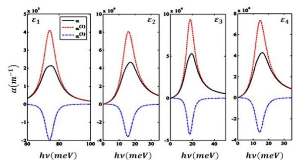
شکل ۱. نمودارهای ضریب جذب خطی، مرتبه سوم غیر خطی و ضریب جذب کلی به صورت تابعی از انرژی فوتون تابشی در حضور ناخالصی هیدروژنی و به ازای توابع استتار متفاوت، L = 8 nm و x = 0.3 .
