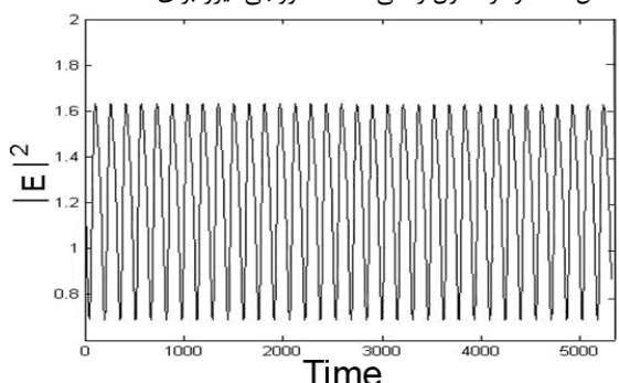
شکل ۵: نمودار تحول زمانی شدت خروجی لیزر برای kl = 0.2 .
