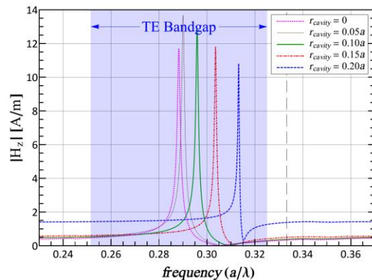
شکل ۲: اندازه مولفه z میدان مغناطیسی در نقطه ای نزدیک به کاواک و در صفحه میانی تیغه بر حسب فرکانس برای کاواک ها با شعاع مختلف. ناحیه آبی رنگ بیانگر گاف بلور پایه است
