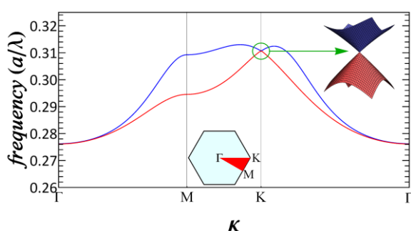
شکل ۴: دو باند محاسبه شده از روش تنگ بست
