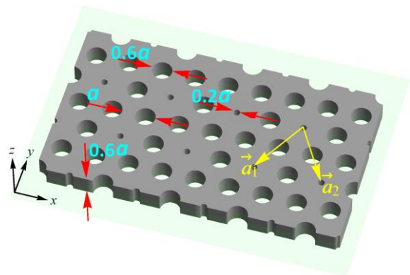
شکل ۳: ابر بلور طراحی شده که ساختار باند آن دارای نقطه دیراک است
