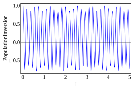
شکل ۳: وارونی جمعیت برحسب زمان مشخصه \tau = \lambda_1 t به ازای p = 100, \zeta = 3, \gamma_1 = 1, \gamma_i (i = 2, \dots, 6) = 0 .
