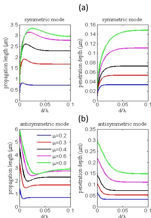
شکل ۳: طول انتشار و جایگزینی (a) مد مقارن (b) مد پادمقارن. \lambda=10\text{ }\mu\text{m} ( \hbar\omega=0.12\text{ eV} ) در نظر گرفته شده است.
