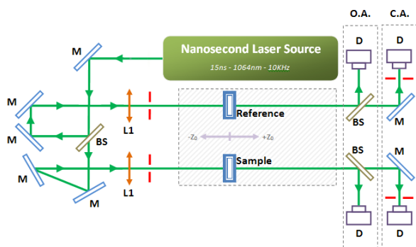
شکل ۱: نقشه شماتیک چیدمان جاروب-Z دوبازویی مورد استفاده. M: آینه بازتاب کامل، BS: تقسیم کننده پرتو، L: لنز (f=300mm)، D: آشکارساز، OA: هندسه روزنه باز، CA: هندسه روزنه بسته.
