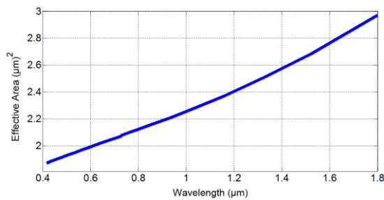
شکل ۲: سطح مقطع موثر بر حسب طول موج برای فیبر شکل ۱.
