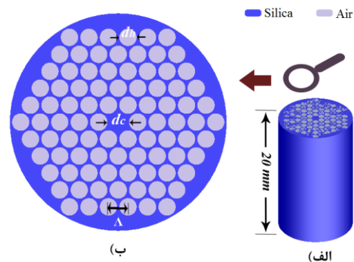
شکل ۴: (الف) فیبر بلور فوتونی به طول ۲۰ میلی‌متر (ب) برش عرضی از سطح مقطع فیبر که حفره‌های هوا با رنگ خاکستری از ماده اصلی تشکیل دهنده فیبر، سیلیکا (رنگ آبی) متمایز شده‌اند و ثابت شبکه‌ای فیبر، \Lambda ، 1.8 \mu\text{m} ، قطر حفره‌های هوا، d_h ، 1.6 \mu\text{m} و قطر هسته فیبر، d_c ، 2 \mu\text{m} هستند.
