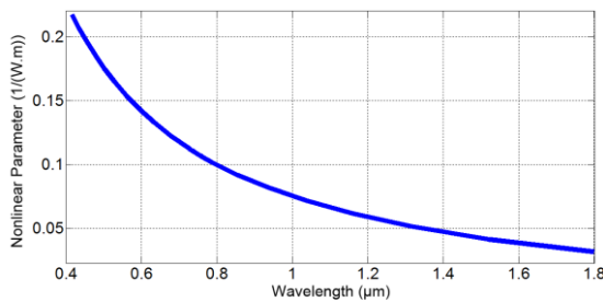
شکل ۳: ضریب غیر خطی بر حسب طول موج برای فیبر شکل ۱.
