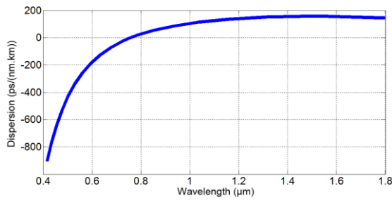
شکل ۱: پاشندگی بر حسب طول موج برای فیبر شکل ۱.
