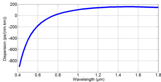
شکل ۱: پاشندگی بر حسب طول موج برای فیبر شکل ۱.
