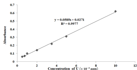
شکل ۲: نمودار تغییرات جذب بر حسب غلظت اورانیم در حجم ۱۰۰ mL از نمونه.
