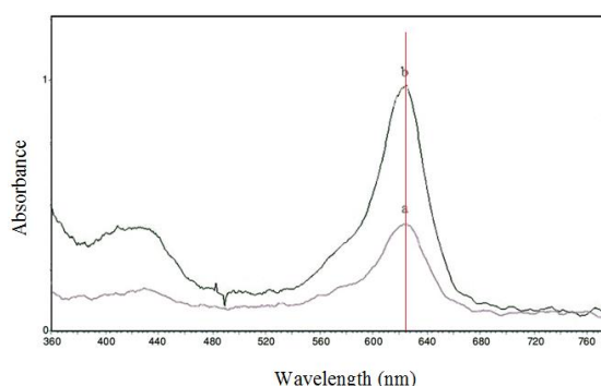
شکل ۱: طیف جذبی برای (a) مالاچیت گرین، (b) زوج یون اورانیم بنزوات با مالاچیت گرین در کلروفرم و اتانول. خط جذب اورانیم در ۶۲۲ nm قرار دارد.
