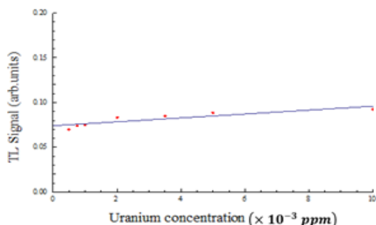
شکل ۵: نمودار کالیبراسیون عدسی گرمایی برای هفت غلظت ۰/۵، ۰/۷۵، ۱، ۲، ۳/۵، ۵ و ۱۰ میکروگرم بر لیتر از ترکیب اورانیوم با مالاچیت گرین.
