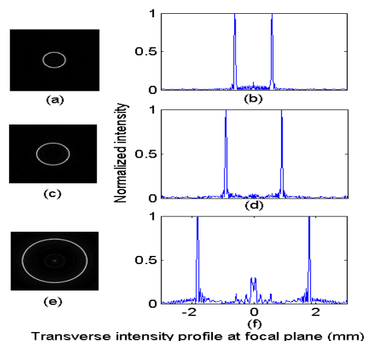
شکل ۱: توزیع شدت عرضی (سمت چپ) و پروفایل شدت (سمت راست) نمونه‌هایی با R=6\text{mm} و \alpha = 0.1, 0.15, 0.3 از بالا به پایین. شعاع حلقه تولیدی نمونه ها به ترتیب ۰.۶mm و ۰.۹ و ۱.۸ است.
