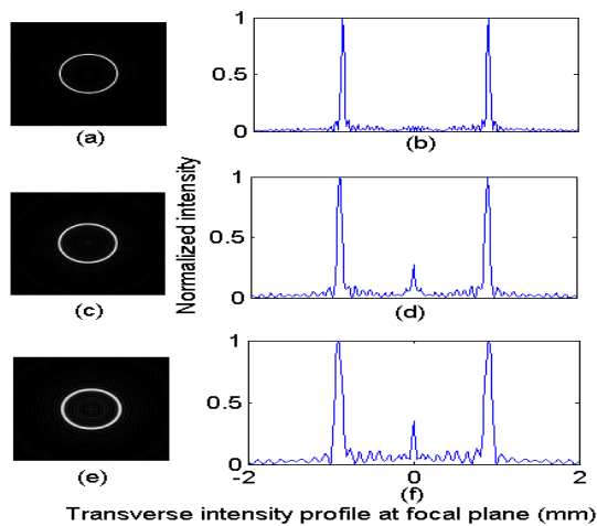
شکل ۲: توزیع شدت عرضی (سمت چپ) و پروفایل شدت (سمت راست) نمونه‌هایی با R=6\text{mm} و \alpha=0.15 و کانونهای f=500 (به ترتیب از بالا به پایین) f=750 , f=1000\text{mm}
