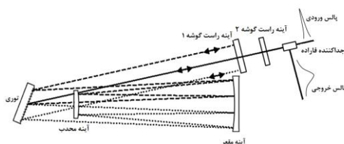
شکل ۱: نمای جانبی پهن‌کننده‌ی آفر دوبار عبور.
