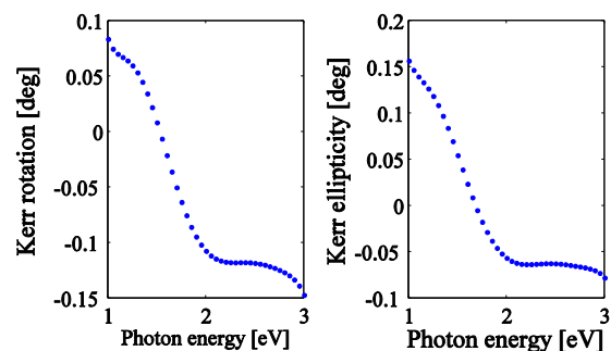
شکل ۳: (چپ) چرخش کر مگنتواینتیکی، (راست) بیضی‌گونگی محاسبه شده توسط روش FDTD بنا شده بر تبدیل Z .
