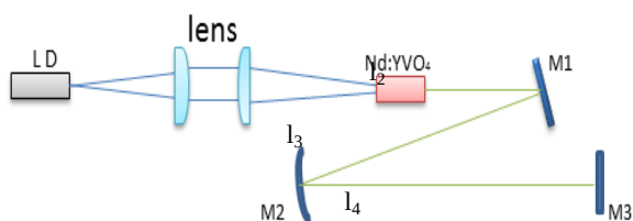
شکل ۱: چیدمان لیزر دمش از انتها Nd:YVO 4
