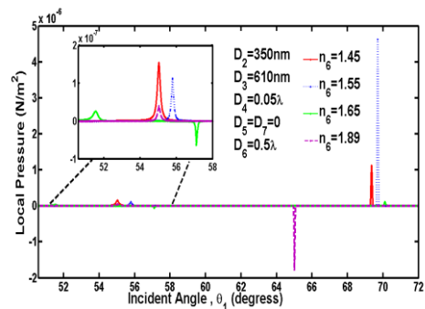
شکل ۳: نمودار فشار اپتیکی وارد بر سلول بر حسب زاویه تابشی بر منشور، برای ساختار شامل سیتوپلاسم‌های با ضریب شکست متغیر با صرف نظر از غشا ( D_5 = D_7 = 0 ).
