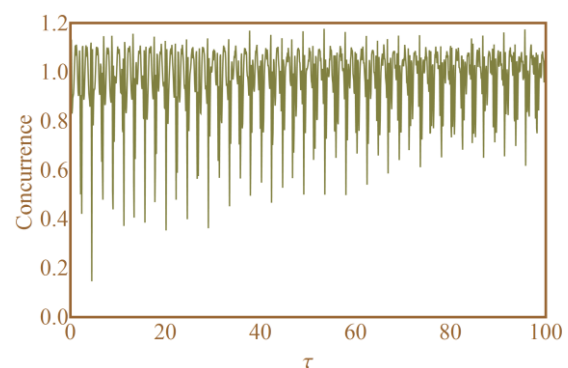
شکل ۳: معیار تلاقی بر حسب پارامتر بدون بعد \tau = gt با پارامترهای مشابه شکل ۱ ولی با |\alpha|^2 = 4 .
