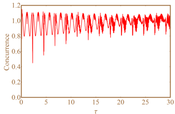
شکل ۲: معیار تلاقی بر حسب پارامتر بدون بعد \tau = gt با پارامترهای مشابه شکل ۱ ولی با \Delta = 15 .
