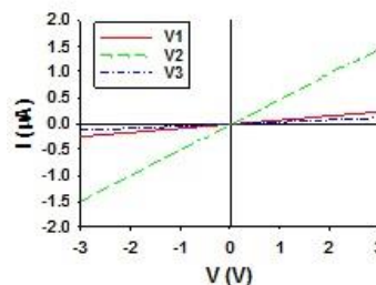
شکل ۷: نمودار جریان-ولتاژ نمونه ها در معرض تابش نور مرئی.
