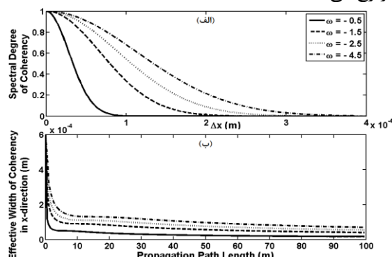
شکل ۲: تغییرات الف) درجه همدوسی در راستای x در z=50m ، ب) عرض مؤثر همدوسی باریکه EPCFT بر حسب فاصله انتشار در اقیانوس متلاطم به ازای قدرت‌های نسبی مختلف نوسانات شوری و دما.
