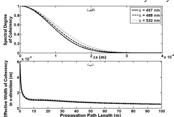
شکل ۳: تغییرات الف) درجه همدوسی در راستای x در z=50m ، ب) عرض مؤثر همدوسی باریکه EPCFT بر حسب فاصله انتشار در اقیانوس متلاطم به ازای طول موج‌های مختلف.
