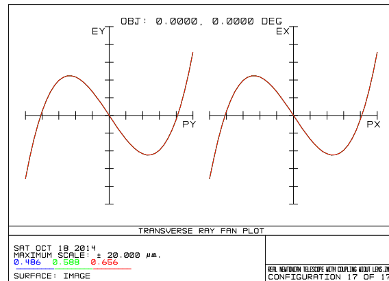
شکل ۵: ابیراهی سیستم در راستای X و Y که توسط نرم افزار zemax برای سیستم فرستنده محاسبه شده است. با ابیراهی حداکثر ۲۰ میکرومتر.
