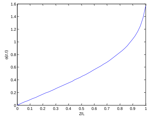
نمودار ۴. تغییرات زاویه‌ی بردار دیرکتور ملکول‌ها بر حسب رادیان
