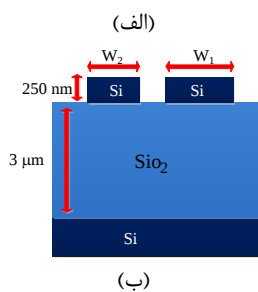
شکل ۱: ساختار فیلتر افزایشی-کاهشی با استفاده از توری‌های براگ ایجاد شده بر روی دیواره موجبرهای نوری: (الف) نمای از بالا (ب) نمای جانبی.
