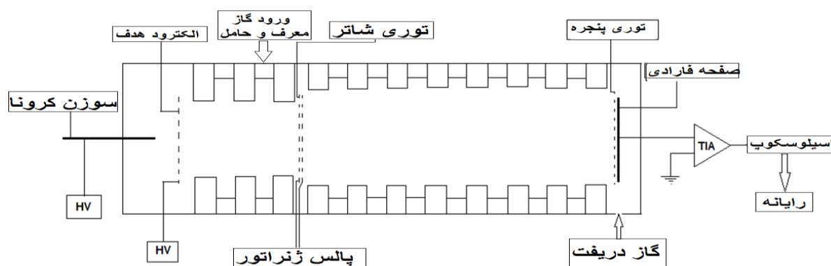
شکل ۱: چیدمان تجربی دستگاه IMS (محل ورود گاز و معرف و حامل مشخص است)
