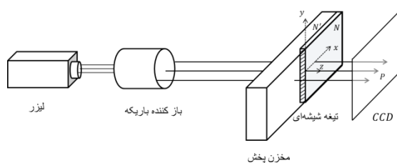
شکل ۱: چیدمان آزمایش اندازه‌گیری ضریب پخش
