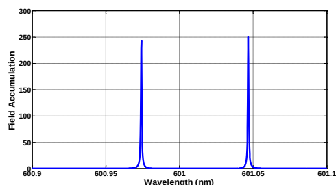
شکل (۸): تشدید بهینه. FWHM = 0.00065 nm, Q \approx 924000
