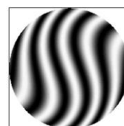
شکل ۶: الگوی تداخلی بیانگر افت کیفیت در سامانه، در نتیجه‌ی ایجاد عدم هم‌مرکزی به میزان DCY=0.1\text{mm} در لنز اول
