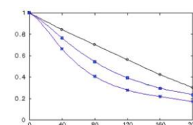
شکل ۱۰: منحنی MTF بیانگر افت کیفیت در سامانه، در نتیجه‌ی ایجاد عدم هم‌راستایی به میزان TLB=0.1^\circ در لنز اول
