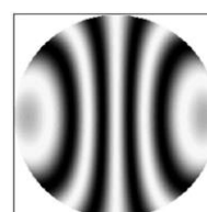
شکل ۹: الگوی تداخلی بیانگر افت کیفیت در سامانه، در نتیجه‌ی ایجاد عدم هم‌راستایی به میزان TLB=0.1^\circ در لنز اول
