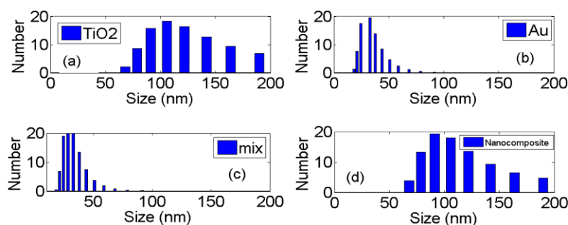
شکل ۴: توزیع اندازه نانوذرات (a) اکسیدتیتانیوم (b) طلا (c) مخلوط نانوذرات طلا و اکسیدتیتانیوم قبل از تابش لیزر (d) نانوکامپوزیت (آلیاژ) نانوذرات طلا و اکسیدتیتانیوم.
