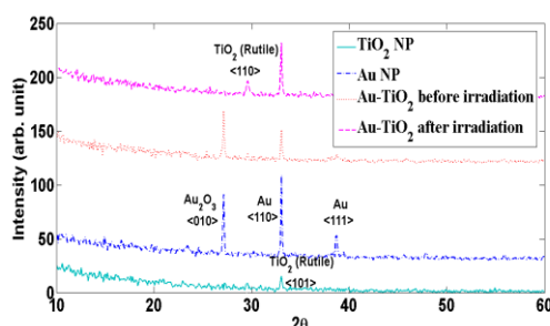
شکل ۳: طیف پراش اشعه X نمونه های نانوذرات طلا و اکسید تیتانیوم به همراه طیف مخلوط آنها قبل و بعد از تابش لیزر ۵۳۲ نانومتر.
