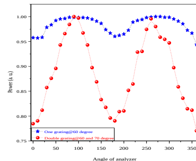
شکل ۳: پاسخ قطبشگرهای فلزی به تفکیک یک قطبشگر با زاویه ۶۰ درجه (مثلث) و دو قطبشگر متصل به هم با زوایای ۶۰ و ۷۰ درجه (دایره).
