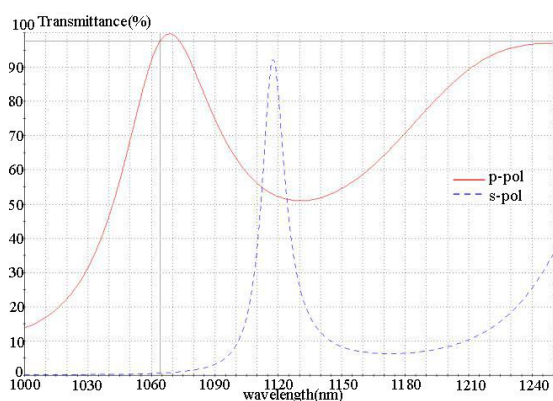
شکل ۱: نمودار تراگسیل قطببنده طراحی شده که توسط نرم افزار طراحی لایه‌های نازک رسم شده است.
