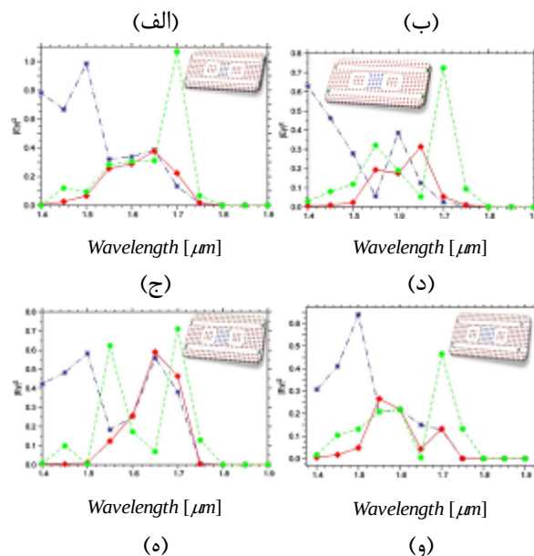
شکل ۴: پاسخ طیفی توان انتقالی ساختار تشدیدگر حلقوی دوتایی بر بلور فوتونی در هندسه موازی، نمودار خط‌پر (کانال C)، خط تیره (کانال D) و خط تیره - دو نقطه (کانال B)
