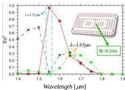
شکل ۵: بررسی تاثیر تغییر شعاع میله‌های توزیع‌گر بر روی پاسخ طیفی توان انتقالی تشدیدگر حلقوی دوتایی بلور فوتونی در هندسه موازی
