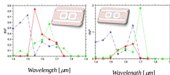
شکل ۵: بررسی تاثیر تغییر شعاع میله‌های تزویج‌گر بر روی پاسخ طیفی توان انتقالی تشدیدگر حلقوی دوتایی بلور فوتونی در هندسه موازی
